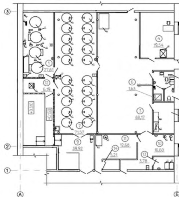
Схема расположения оборудования
